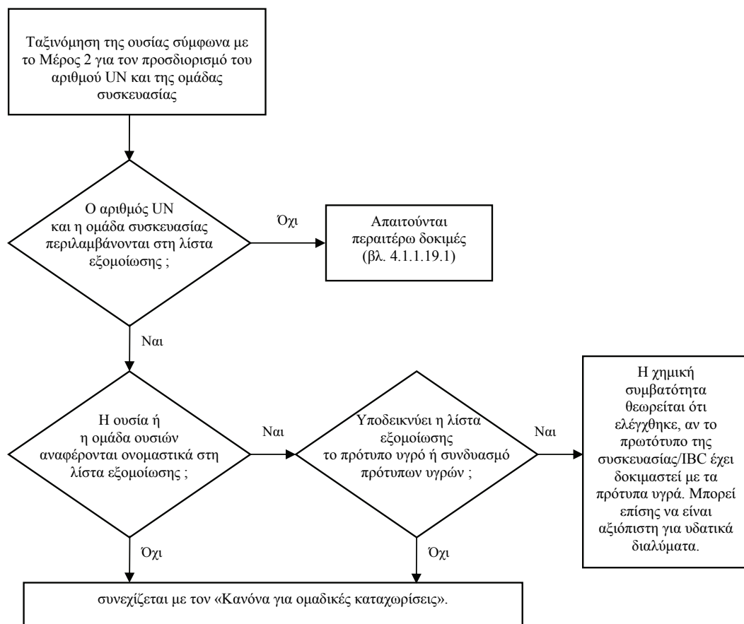
Σχήμα 4.1.1.21.1. Διάγραμμα για την εξομοίωση της πληρωτικής ουσίας με πρότυπα υγρά.
