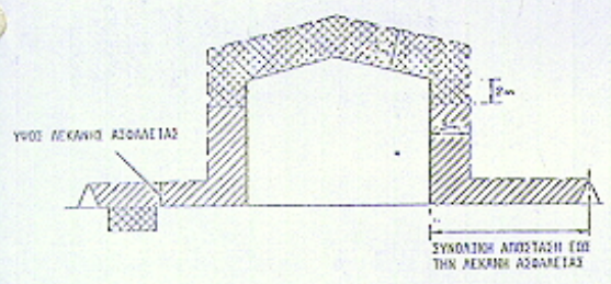
ΔΕΞΑΜΕΝΗ ΜΕ ΚΥΚΛΙΚΗ ΟΡΟΦΗ
