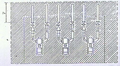
ΑΡΙΘΜΑ ΠΥΛΩΝ ΚΑΙ ΜΗΤΡΩΠΕΣ ΚΑΤΑΣΚΕΥΗΣ
